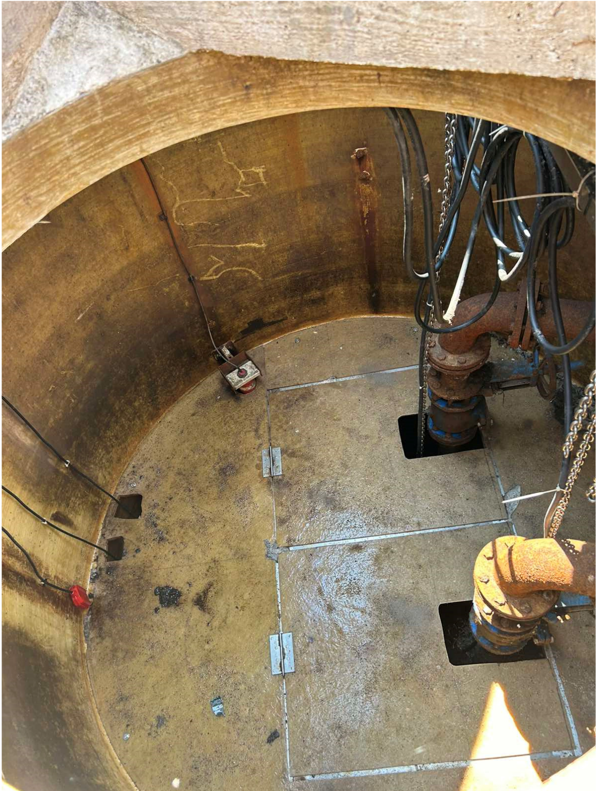
Slika2: Rezervoar iz steklenih vlaken s prikazom priključkov dveh potopnih črpalk
