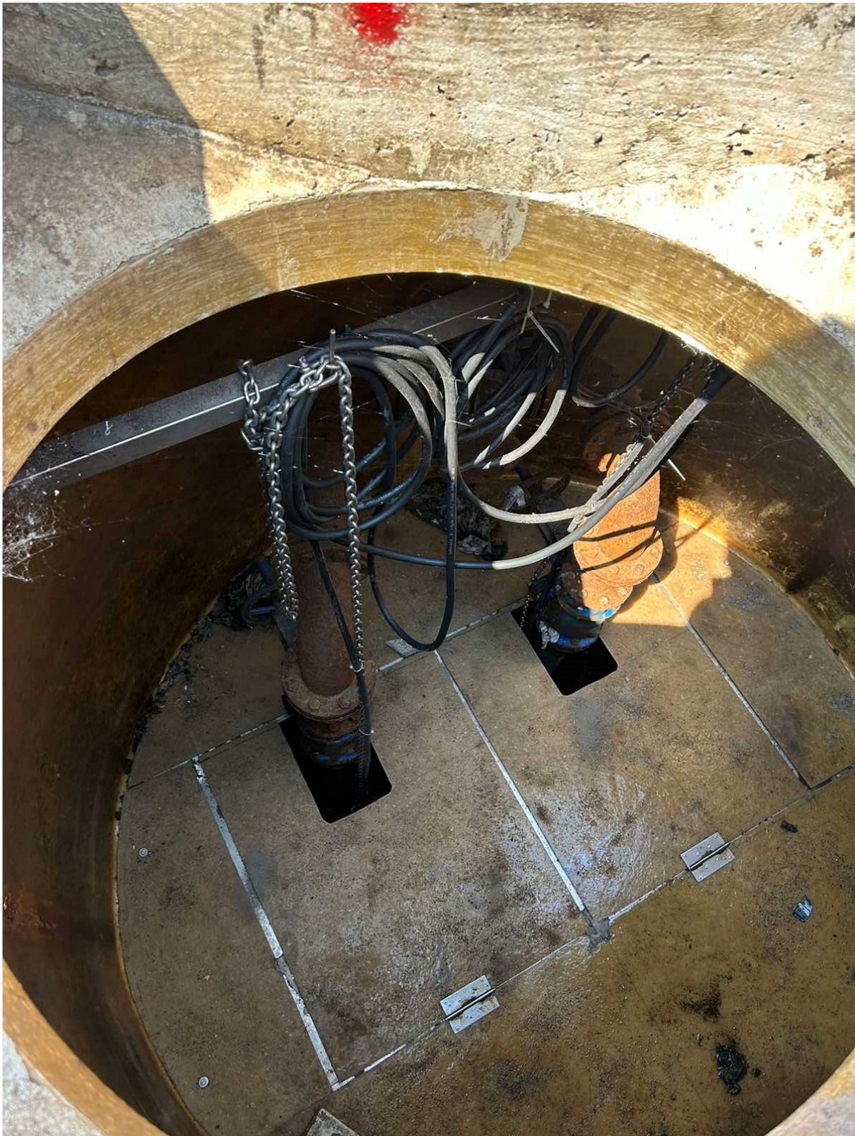
Slika4: Drog za pomoč pri dvigu črpalk (predmet naročila je projektiranje enostavnejšega in bolj varnega načina za dvig črpalk)
