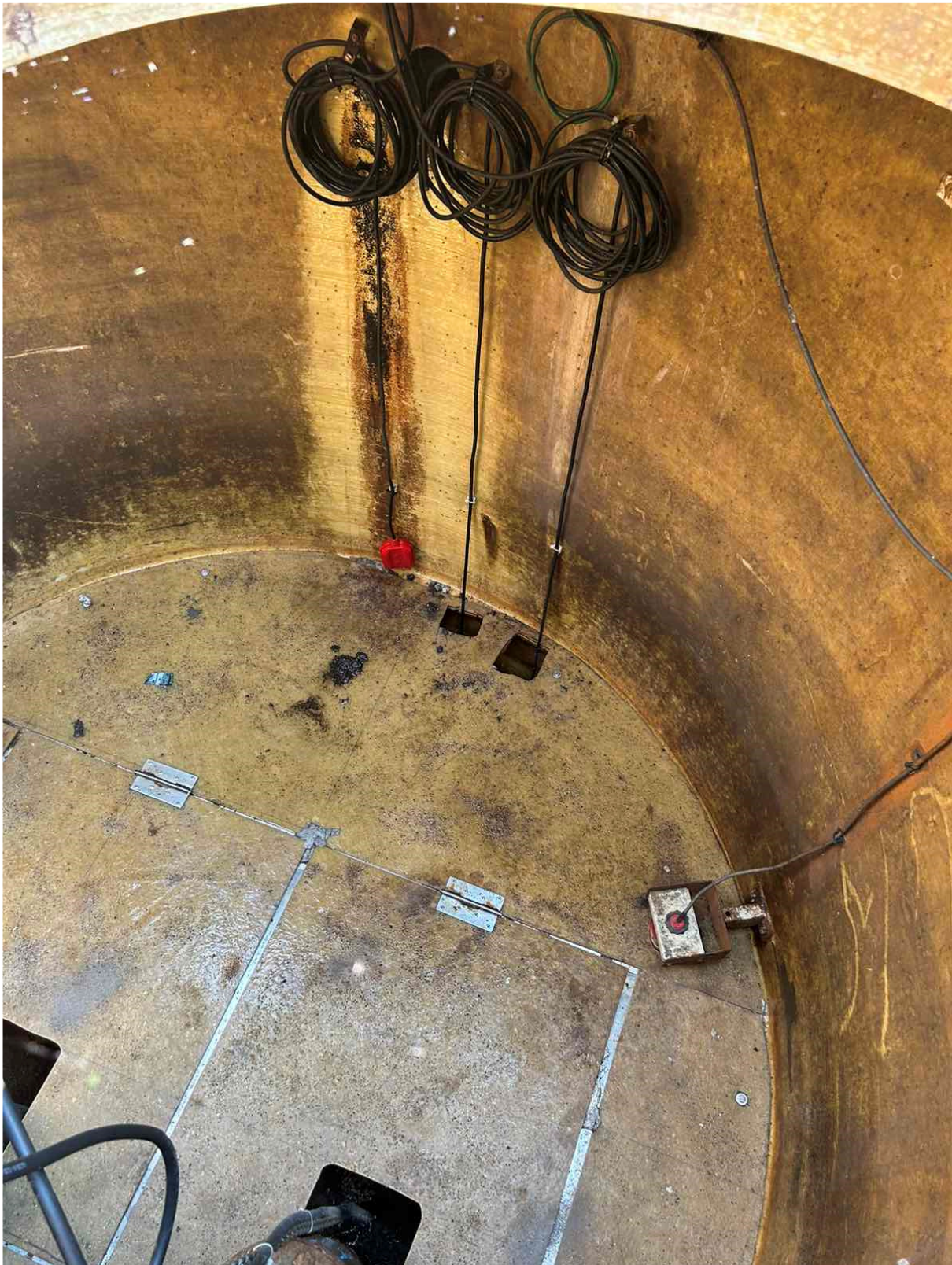
Slika3: Prikaz elektro napajanja črpalk in revizijskih pokrovov na rezervoarju, ki omogočajo dostop do črpalk
