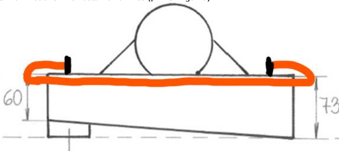
Slika 4: stranski ris nastavka za vilice (primer z gumo)
