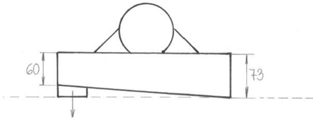
Slika 2: stranski ris nastavka za vilice («copate» pogovorno)
