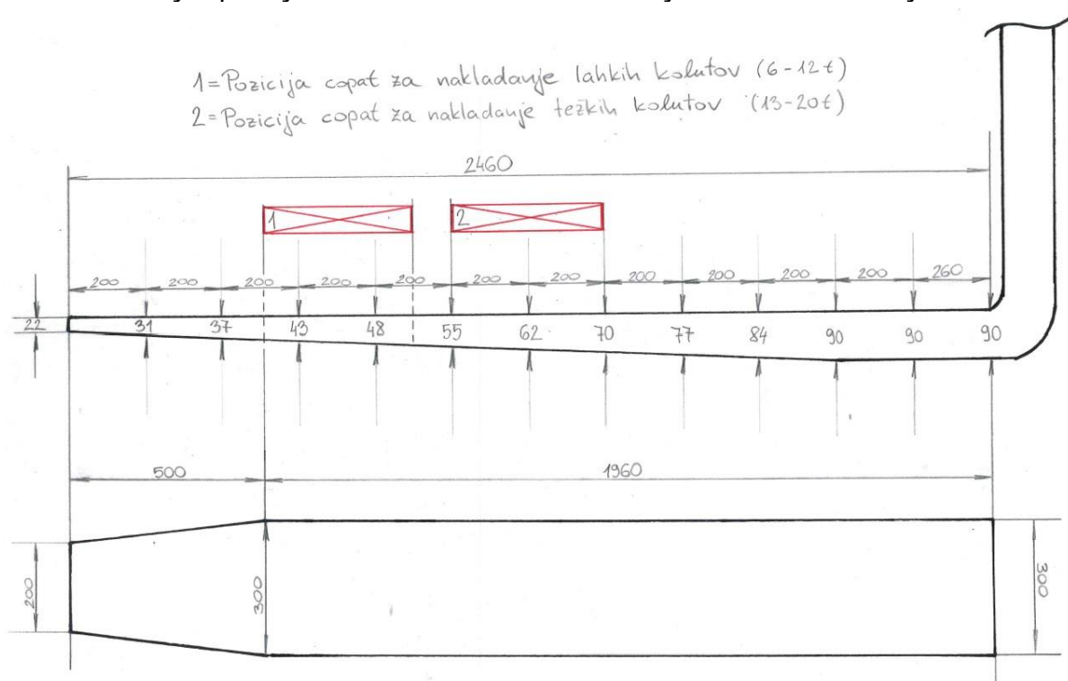
Slika 3: Običajna pozicija nastavka za vilice ob nakladanju in skica vilic viličarja
