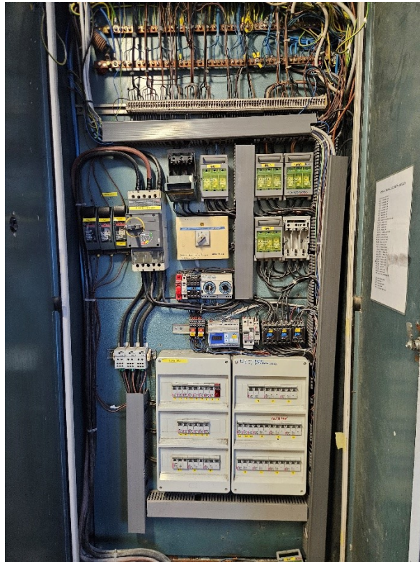
Slika 2: »razdelilna omara«
